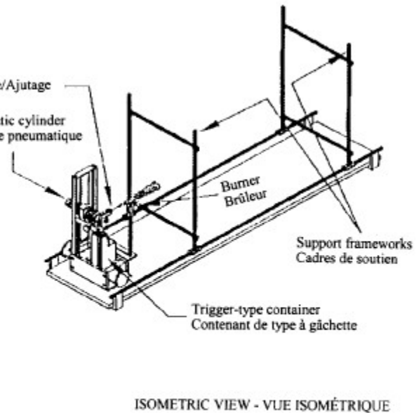
FIGURE 2 Dispositif vérificateur d'inflammabilité Atomiseur
